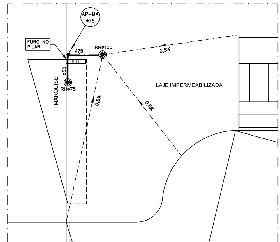
PLANTA BAIXA - COBERTURA DO HALL DE ENTRADA ESCALA 1:100
