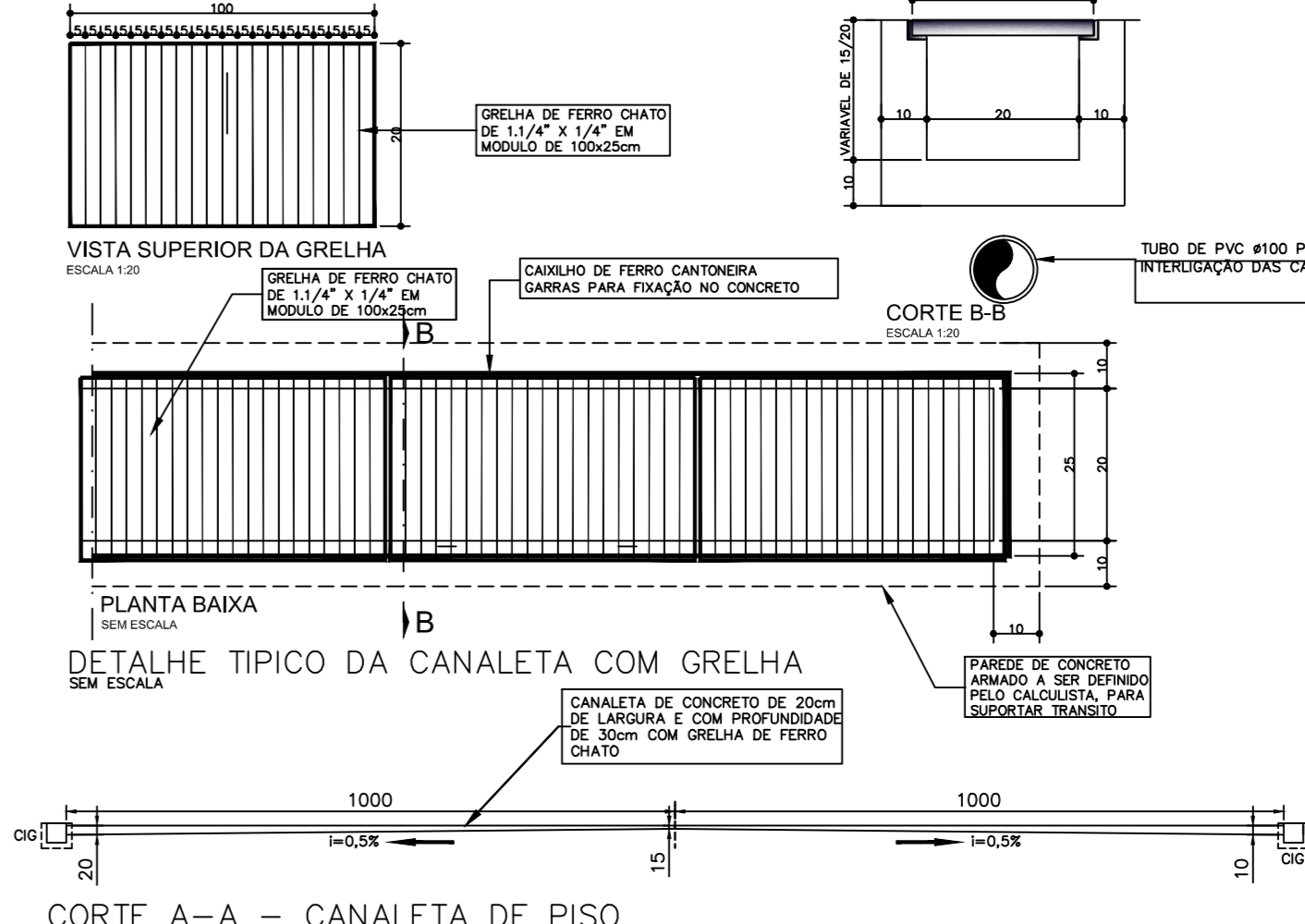
CORTE A-A - CANALETA DE PISO ESCALA 1:100
