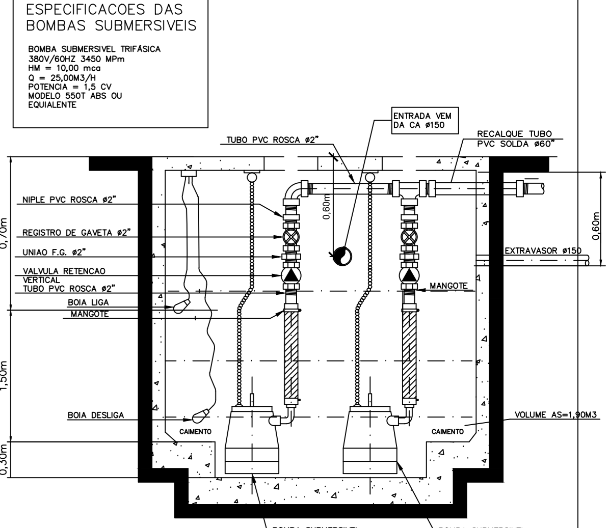
D-BAP DETALHE TÍPICO DAS BOMBAS DE ÁGUA PLUVIAL SEM ESCALA
