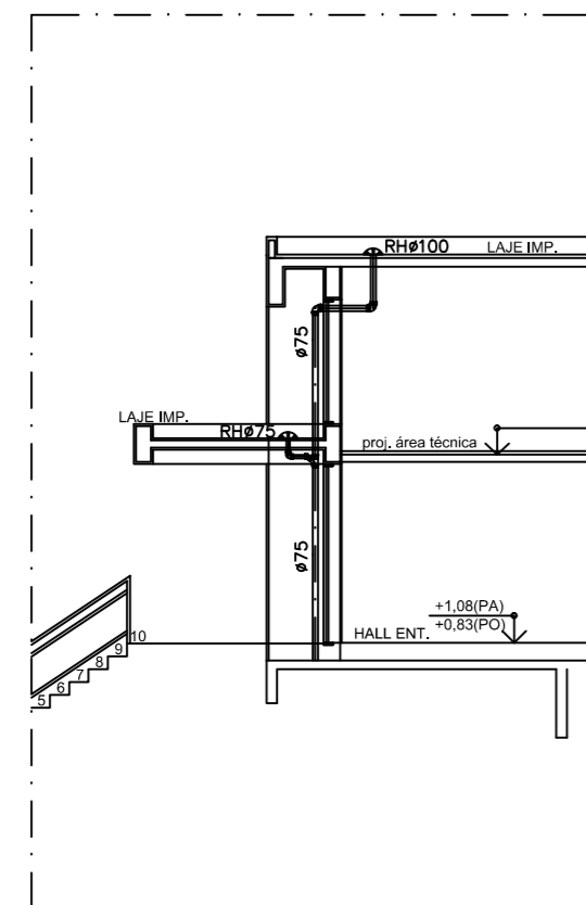
CORTE ESCALA 1:100
