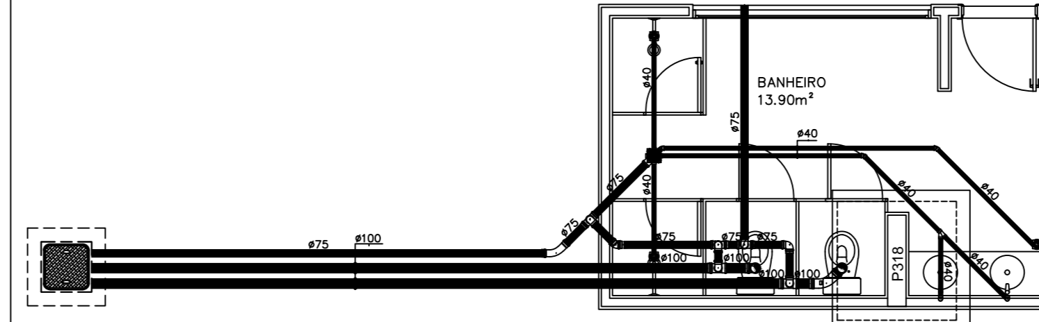
PLANTA BAIXA - DETALHE 3 ESCALA 1:100
