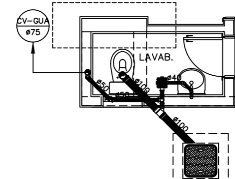
PLANTA BAIXA - DETALHE 1 ESCALA 1:100
