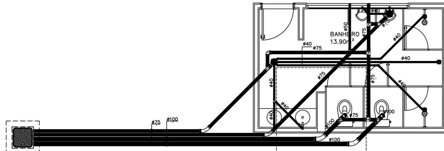
PLANTA BAIXA - DETALHE 2 ESCALA 1:100
